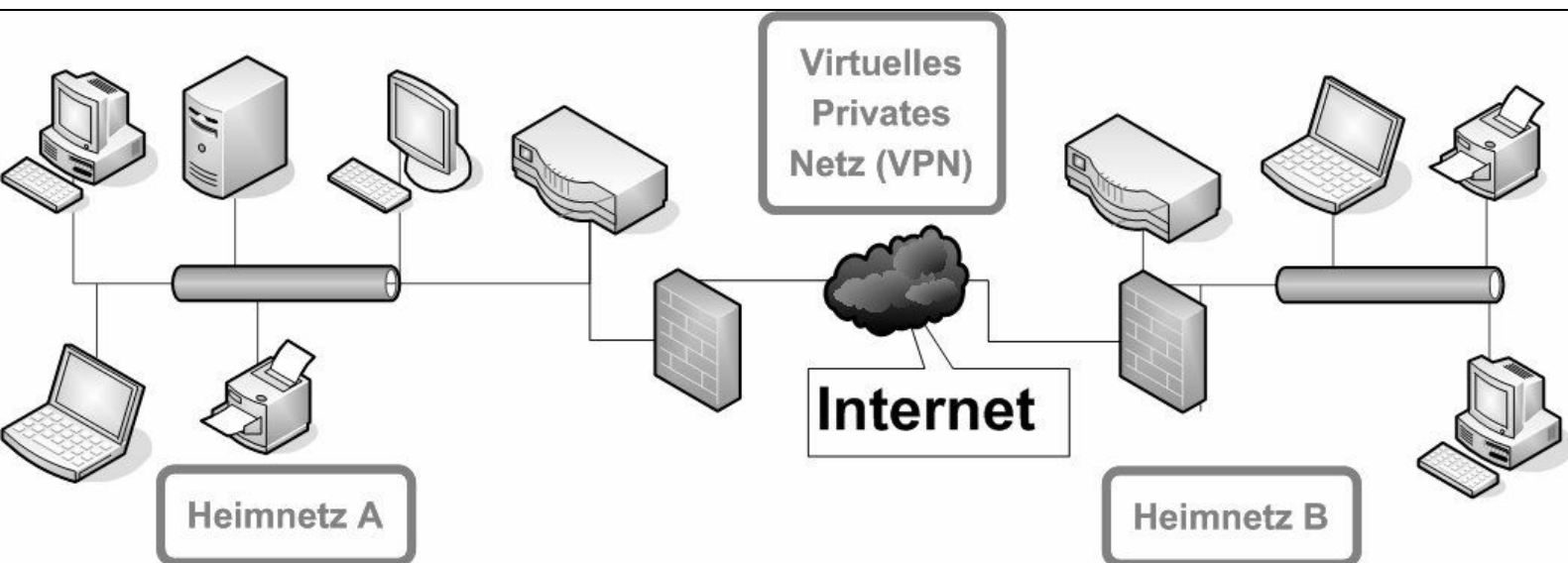
Bild 8.12 Sind zwei Netzwerke miteinander verbunden, können sämtliche Geräte aus Heimnetz A auf alle Geräte in Heimnetz B zugreifen. Damit lassen sich – abhängig von der DSL-Up- und -Downstream-Geschwindigkeit – Daten hin- und hertransferieren, gemeinsame Musik- und Videobestände nutzen und vieles mehr.
