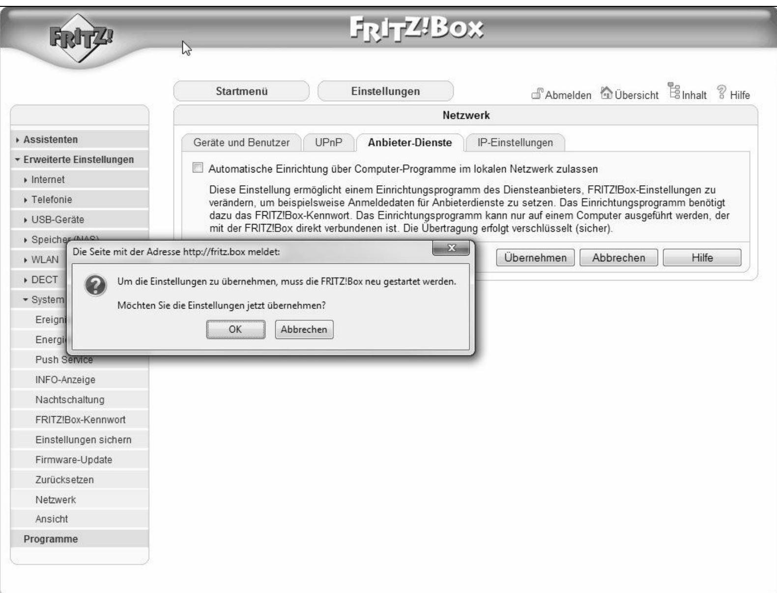
Bild 3.21 Nachdem das Häkchen entfernt wurde, fordert die FRITZ!Box einen Neustart der Anlage an, was weniger als zwei Minuten dauert.
